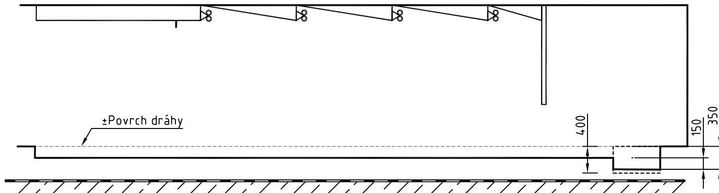
C. Usporiadanie pre nízky rošt - zapustený - dráhy a dopadište zapustené v podlahe
