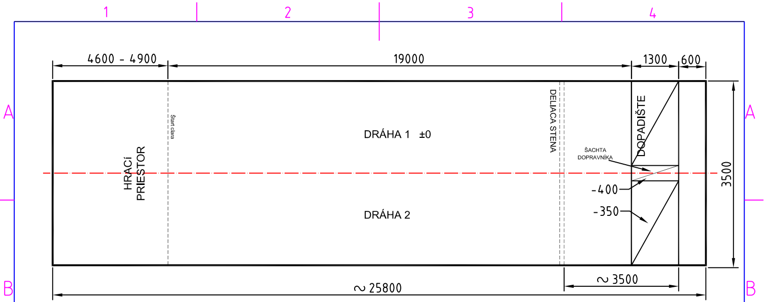
A. Usporiadanie pre vysoký rošt dráhy a dopadište umiestnené nad úrovňou podlahy
