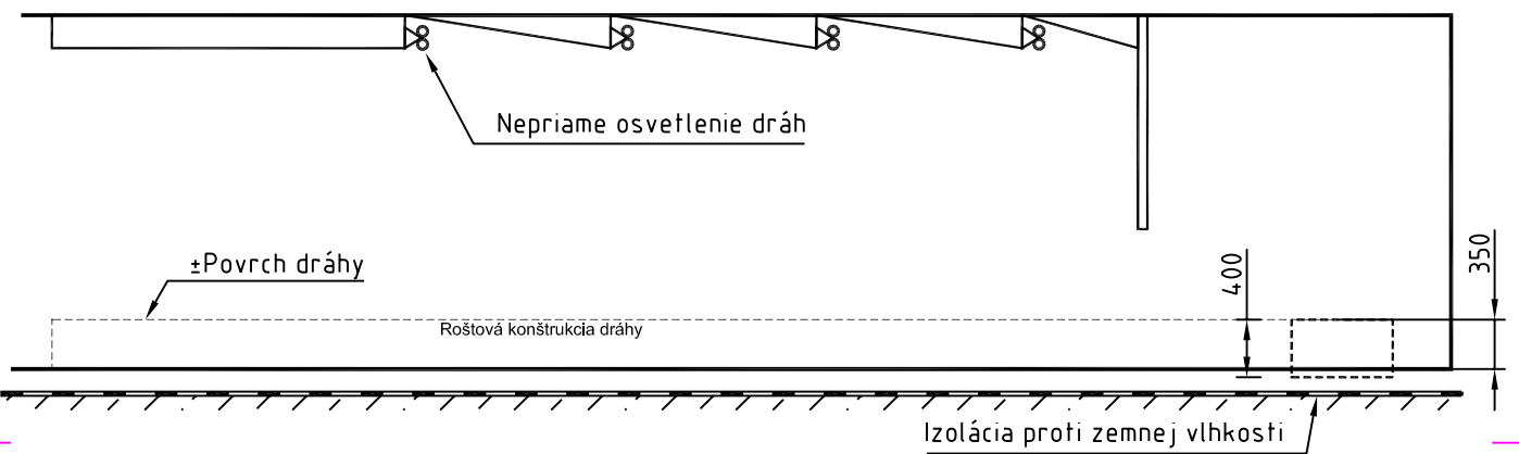
B. Usporiadane pre nízky rošt - dopadište zapustené v podlahe
